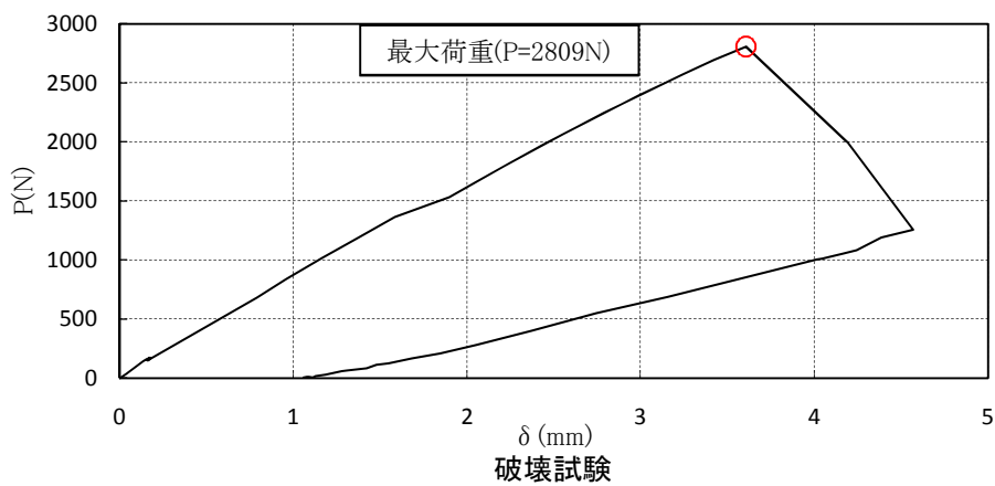
図-1 P- \delta 関係
